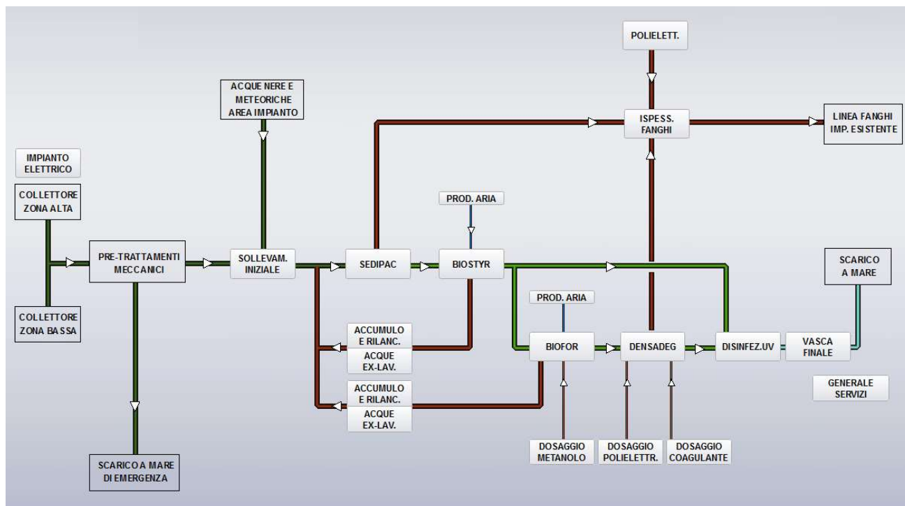
FIGURA 17 - SCHEMA FLUSSO DEPURATORE DI SERVOLA
