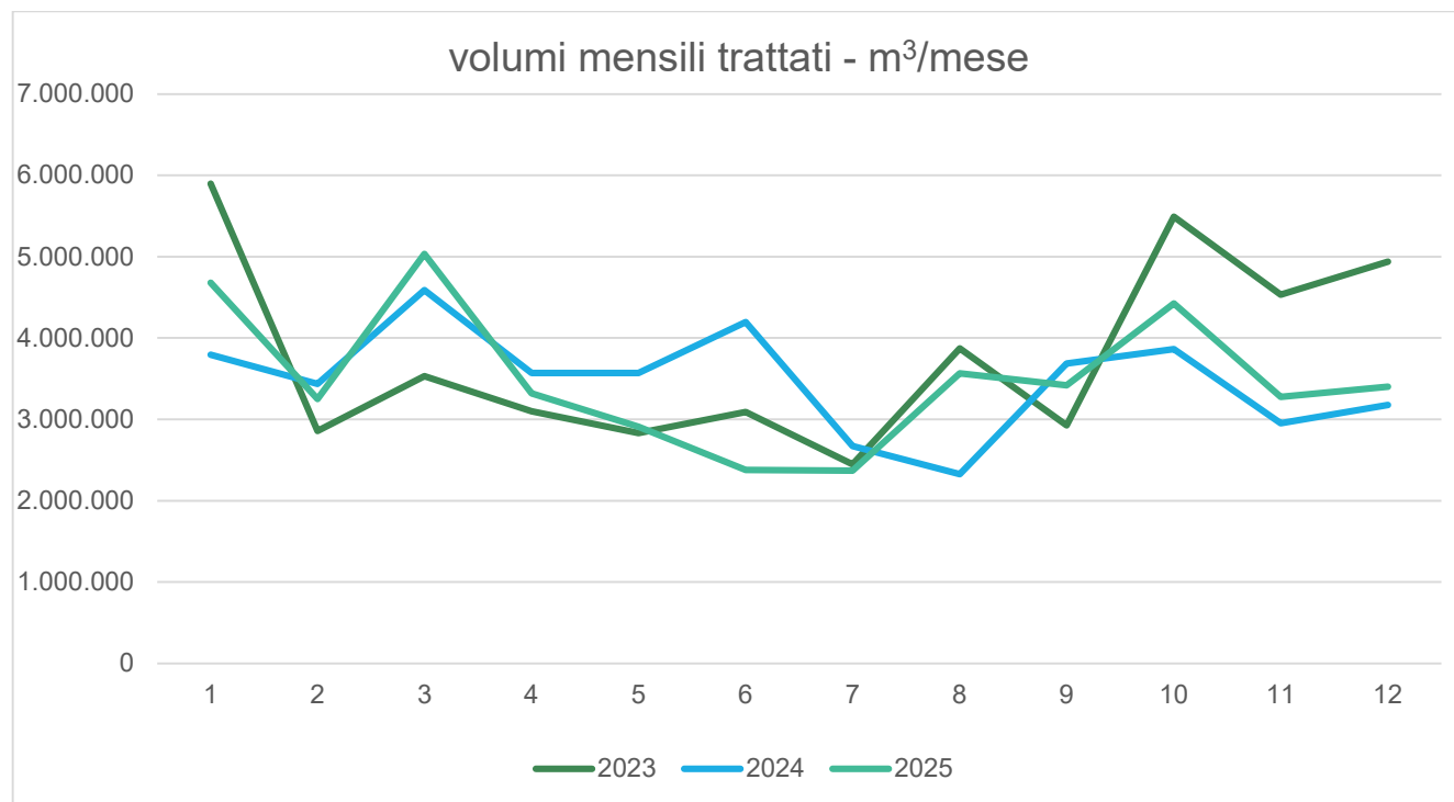
FIGURA 20 – VOLUMI MENSILI TRATTATI DALL'IMPIANTO DI DEPURAZIONE DI SERVOLA
