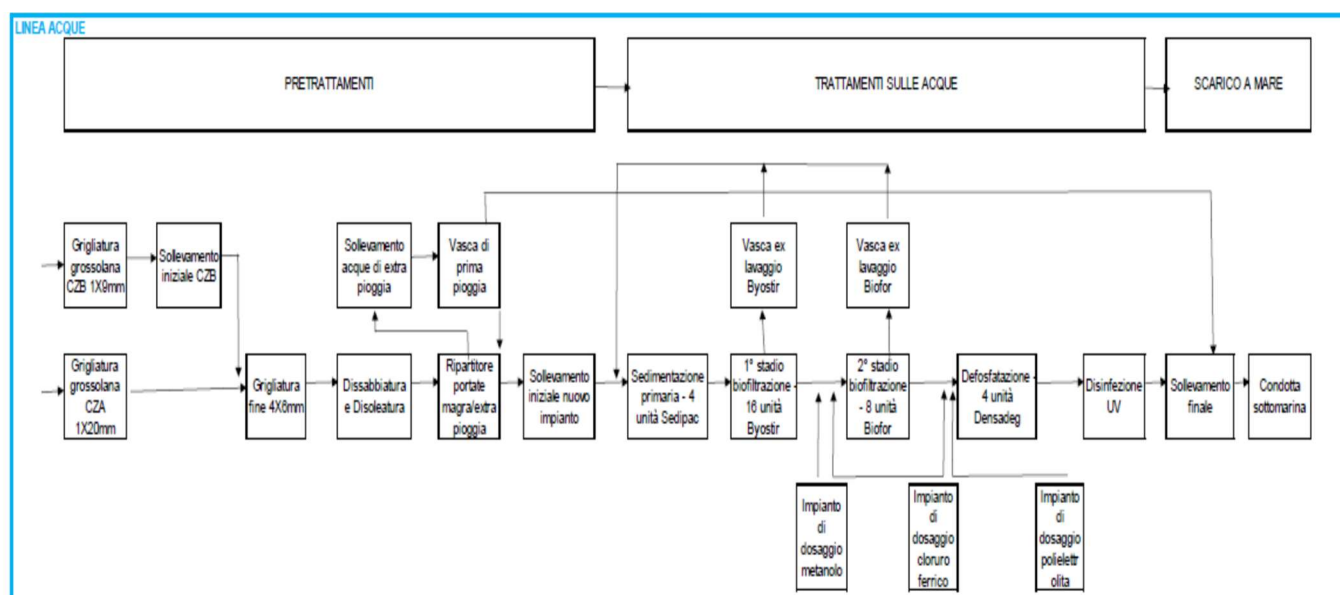
FIGURA 18 – SCHEMA DI FLUSSO LINEA ACQUA
