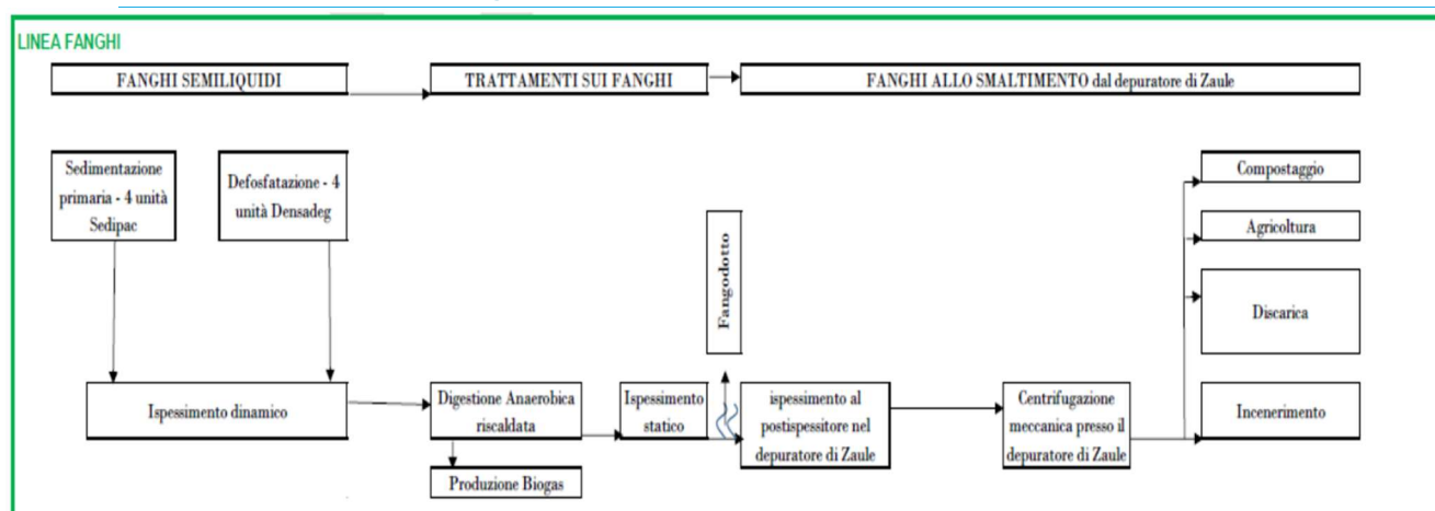
FIGURA 19 – SCHEMA DI FLUSSO LINEA FANGHI
